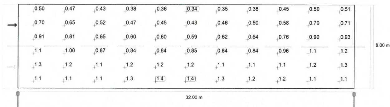
Observator 2: Valoarea de întreținere, densitatea luminii cu carosabil uscat [ \text{cd}/\text{m}^2 ] (Raster valoric)
