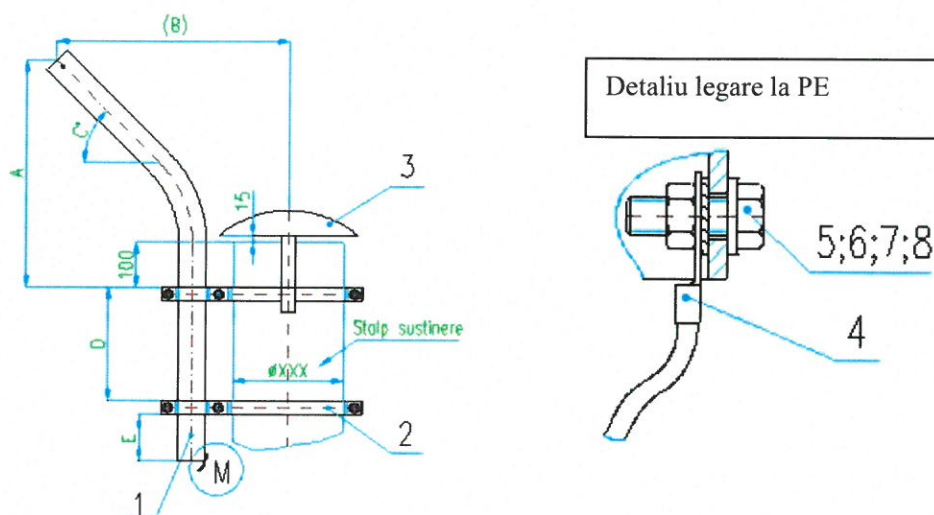
Fig.1-montarea consolei cu coliere pe stâlp:
